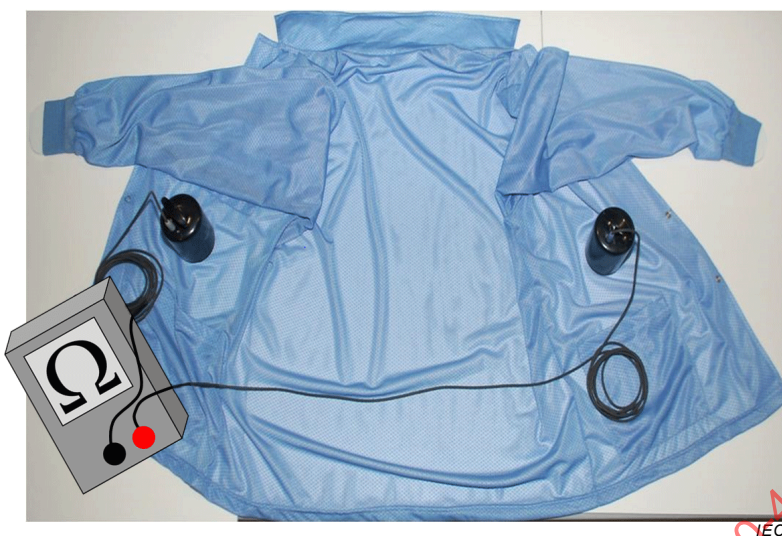
Figure 3 – Montage d'essai – Résistance point à point (procédure pièce à pièce avec surface de support isolante)
