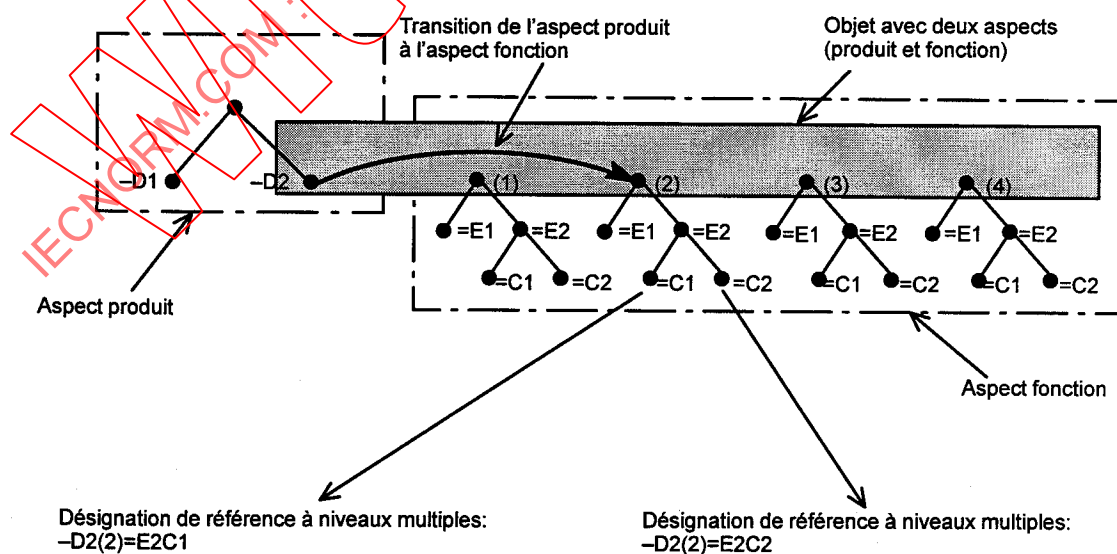
Figure 26 - Exemple de désignations de référence à niveaux multiples utilisant différents aspects d'un objet avec plusieurs représentations indépendantes dans un aspect unique
