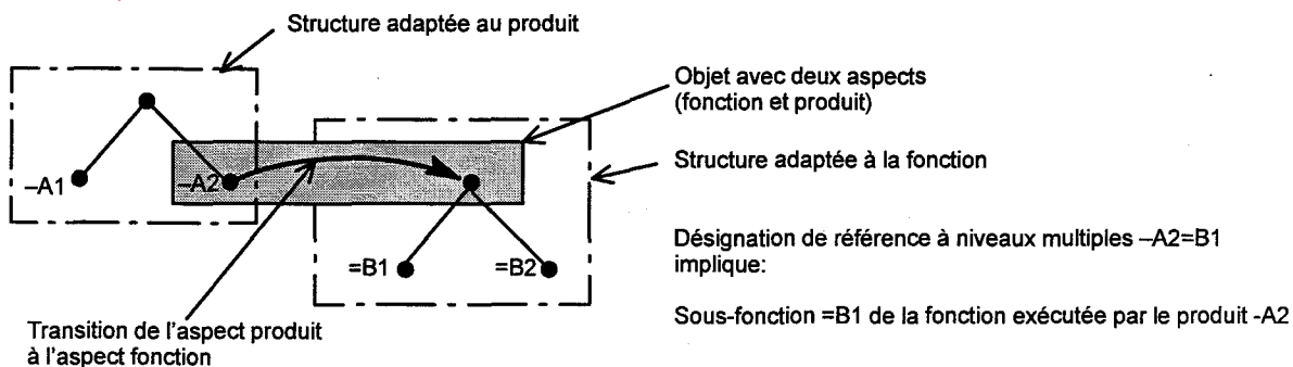
Figure 28 - Transition de l'aspect produit à l'aspect fonction
