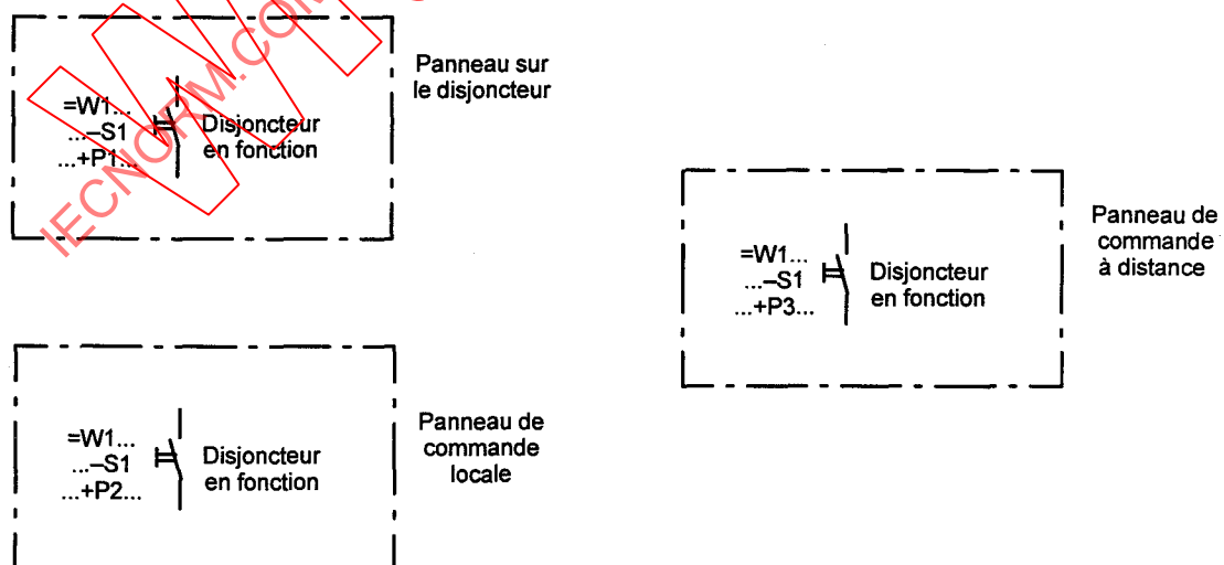
Figure 33 - Exemples de groupes de désignations de référence
