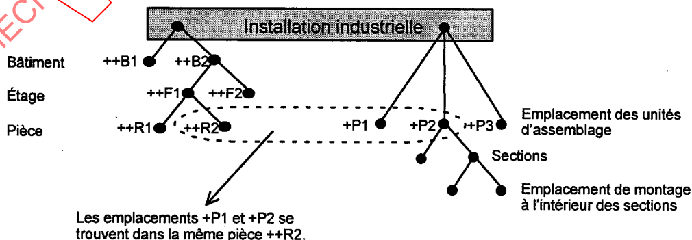
Figure 23 - Structures adaptées à l'emplacement de l'installation industrielle
