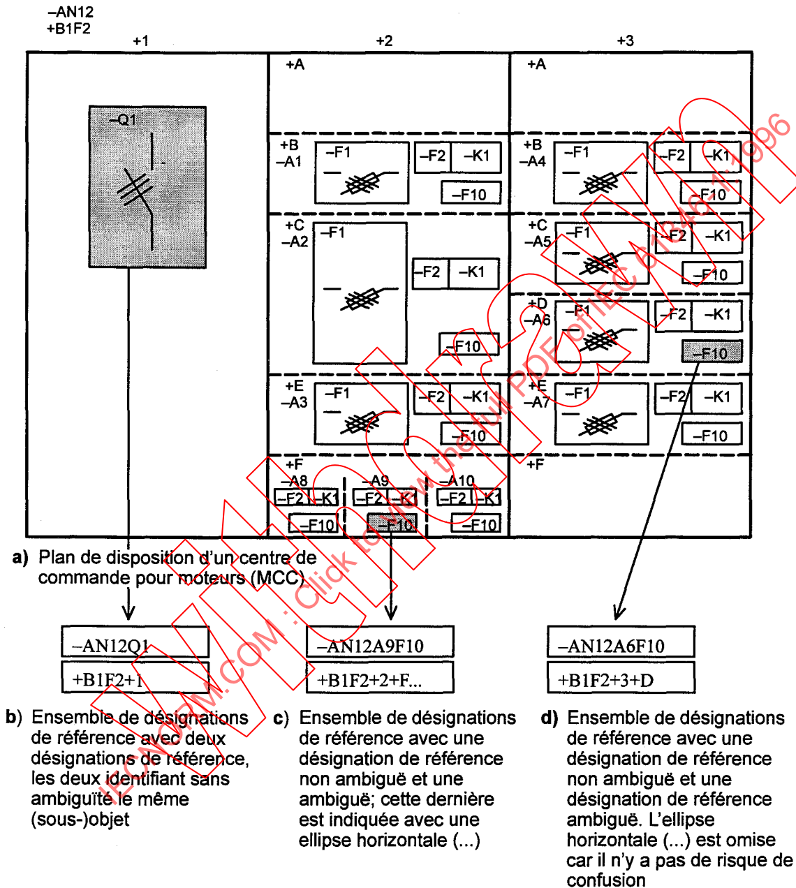
Figure 32 - Exemple d'ensemble de désignations de référence
