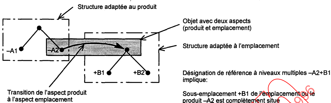
Figure 29 - Transition de l'aspect produit à l'aspect emplacement
