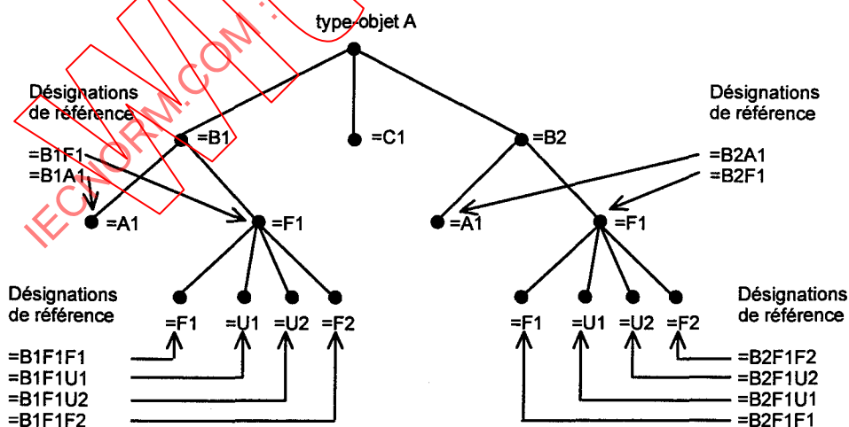
Figure 17 - Structure arborescente adaptée à la fonction concaténée du type-objet A
