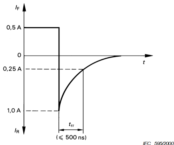
Figure 4c – Temps de recouvrement t_{rr} de la diode
