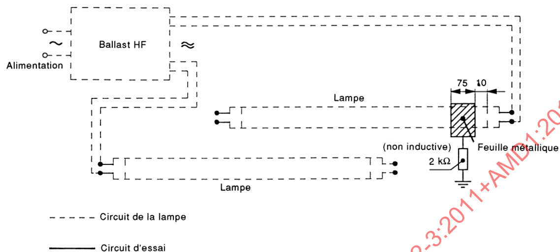
Figure I.1a – Montage d'essai pour les lampes fluorescentes tubulaires en forme de barre
