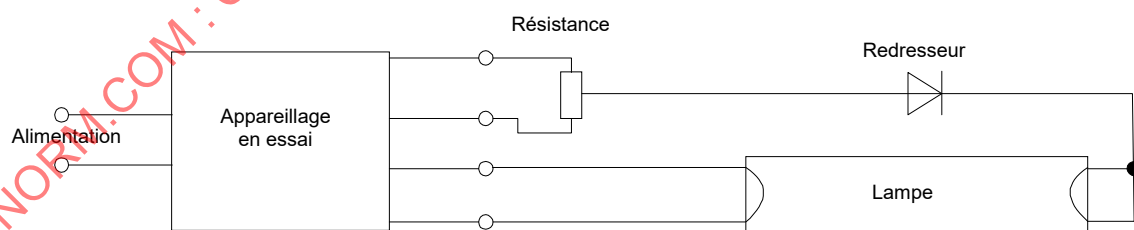
Figure 4b – Essai de la direction opposée de l'effet redresseur
