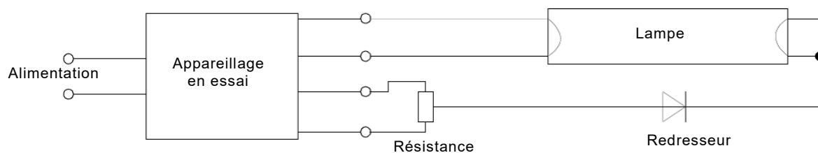
a) Essai du premier sens de l'effet redresseur
