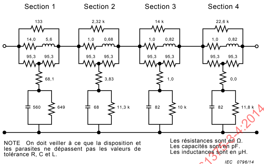
Figure C.3 – Modèle à paire torsadée
