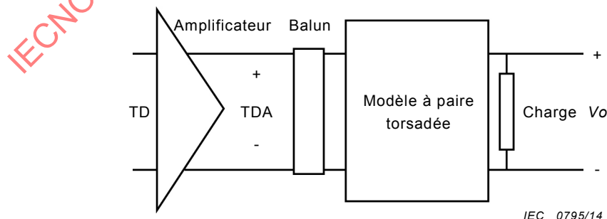
Figure C.2 – Essai de la tension de sortie différentielle
