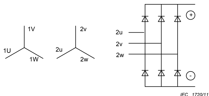
Figure 1 – Montage de double pont hexaphasé B6U ou DB 6
