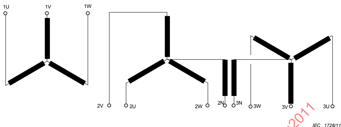
Figure A.2 – Identification des bornes pour couplage d'enroulements Y y0y6
