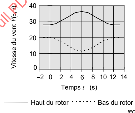
Figure 9 – Exemples de vitesses du vent au niveau des parties supérieure et inférieure du rotor, respectivement, qui illustrent le cisaillement positif transitoire du vent
