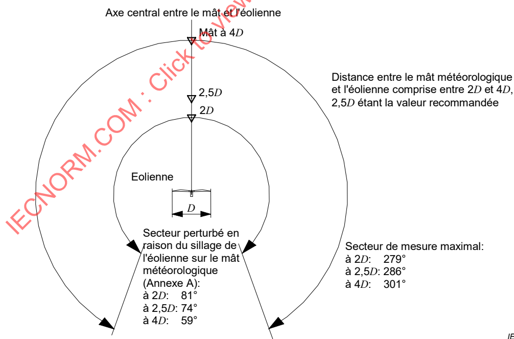
Figure 1 – Exigences de distance entre le matériel de mesure du vent et les secteurs de mesure maximaux admis
