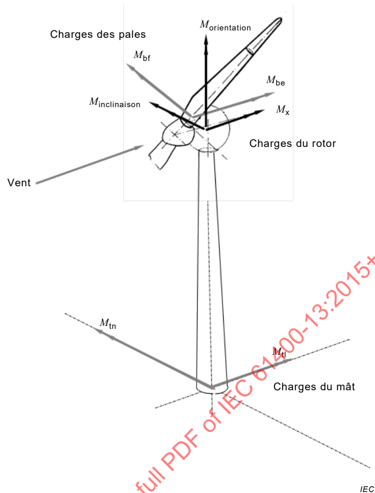
Figure 1 – Charges fondamentales d'une éolienne: charges de la base du mât, du rotor et des pales
