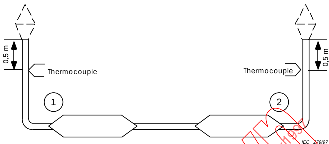
Figure 2 – Jonctions ou dériviées essayées dans l'air
