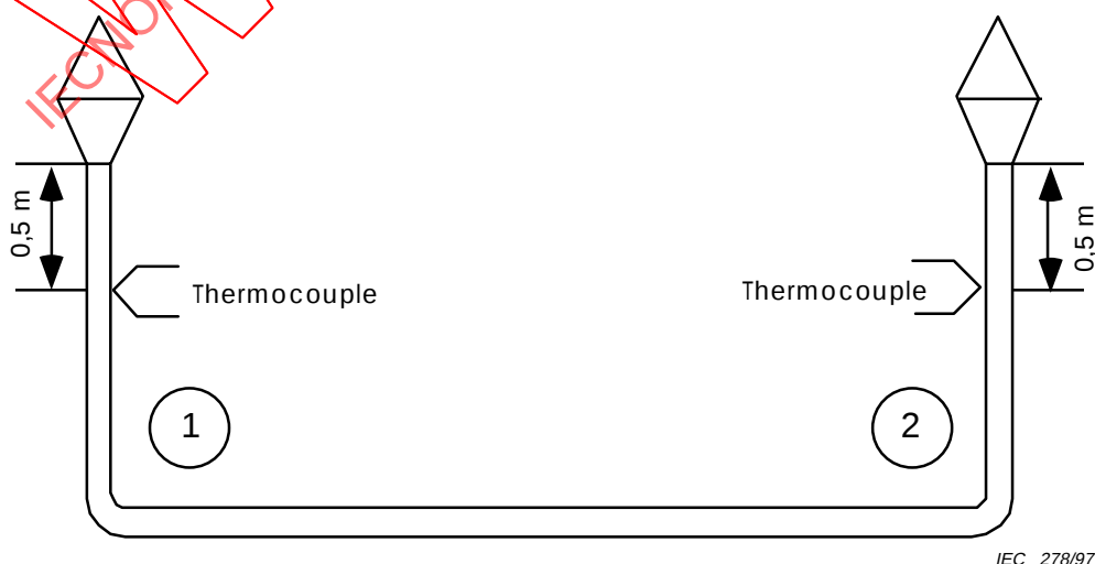
Figure 1 – Extrémités essayées dans l'air
