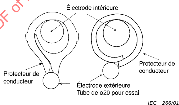
Figure 3a – Disposition de l'électrode extérieure pour essai d'épreuve A2
