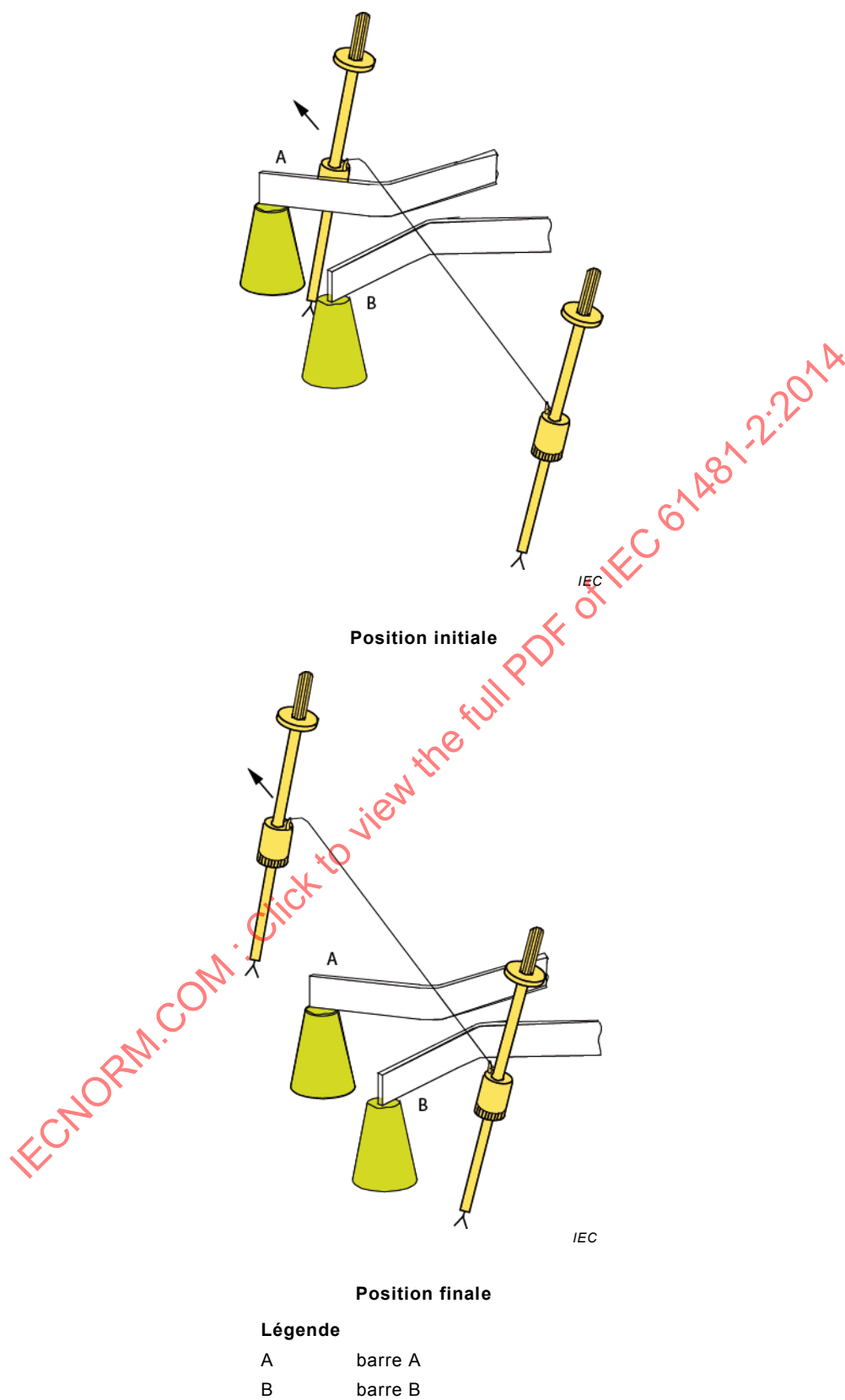
Figure 13 – Essai de contournement du câble de liaison
