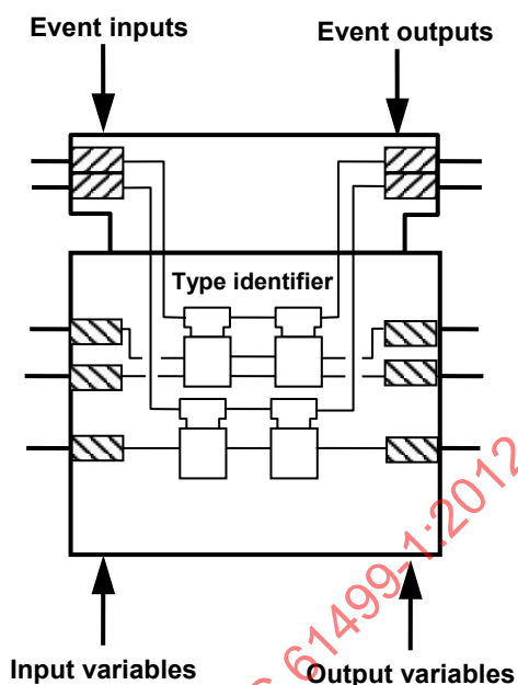
Figure 9b – Bloc fonctionnel composé (5.3)
