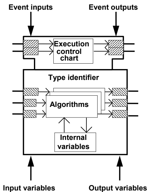
Figure 9a – Bloc fonctionnel de base (5.2)
