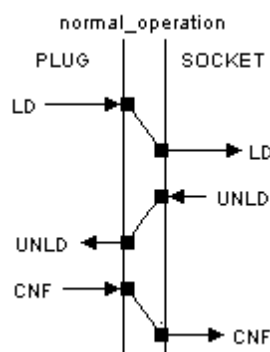
Figure 17b – Séquence de service
