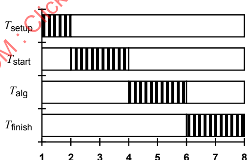
Figure 6 – Modèle d'exécution
