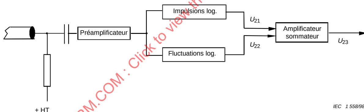
Figure 11 – Schéma d'une chaîne logarithmique à grande dynamique
