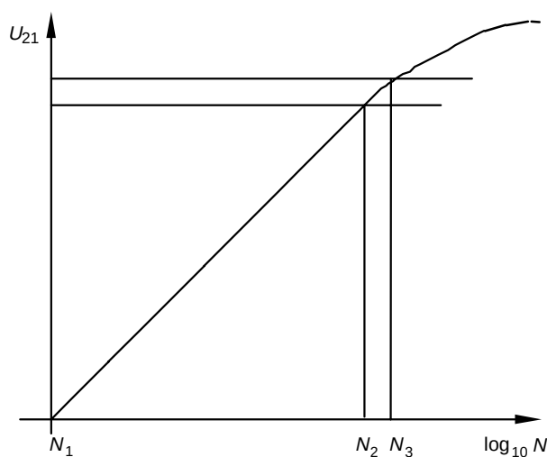
Figure 12a – Réponse du traitement impulsionnel
