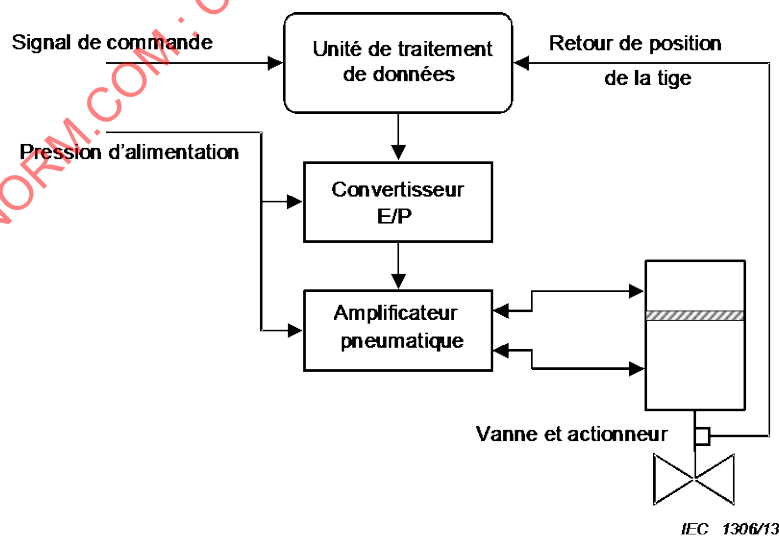
Figure 2 – Conception de base pour des positionneurs à sorties analogiques
