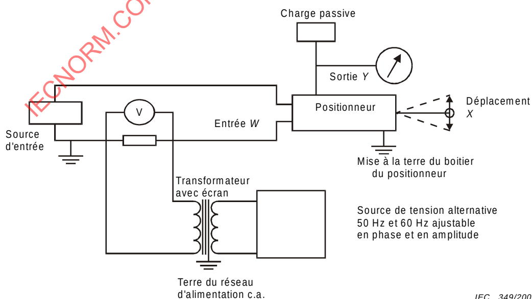
Figure 7 – Perturbations en mode série
