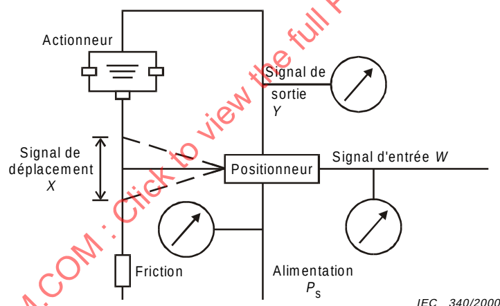
Figure 1a – Positionneur/actionneur à simple effet
