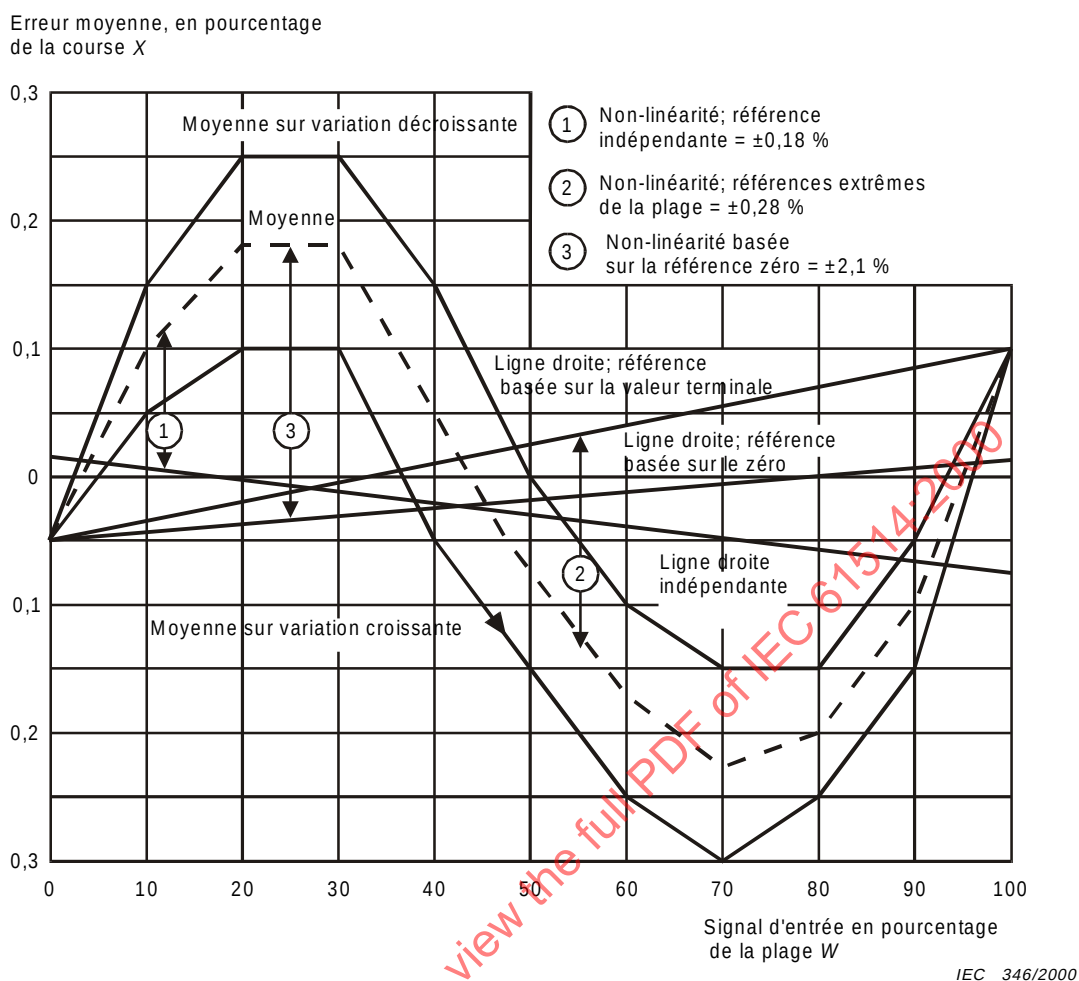
Figure 4 - Courbe typique d'erreurs
