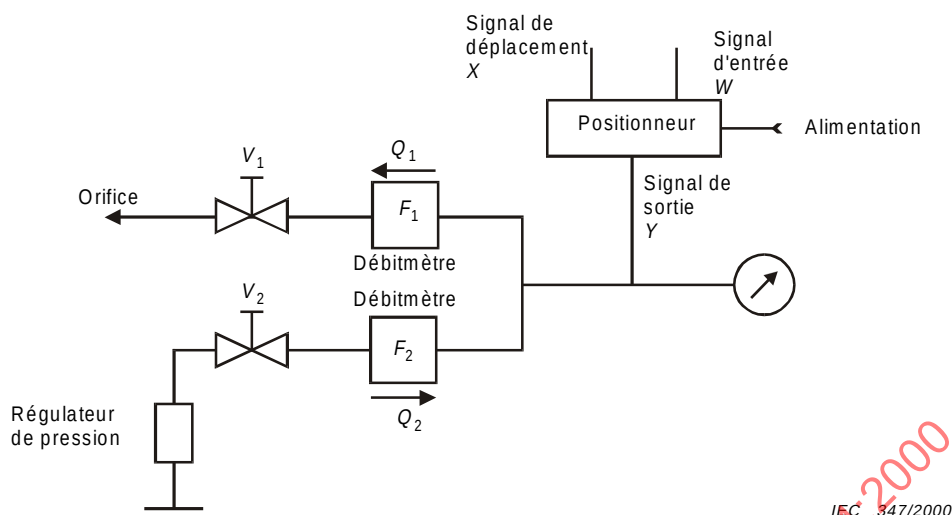
Figure 5 – Dispositions pour les mesures de la caractéristique du débit d'air
