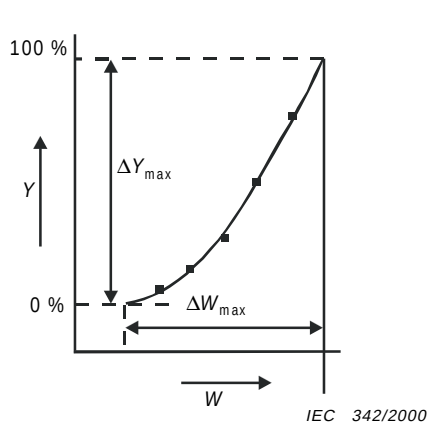
Figure 2a – Positionneur à simple effet
