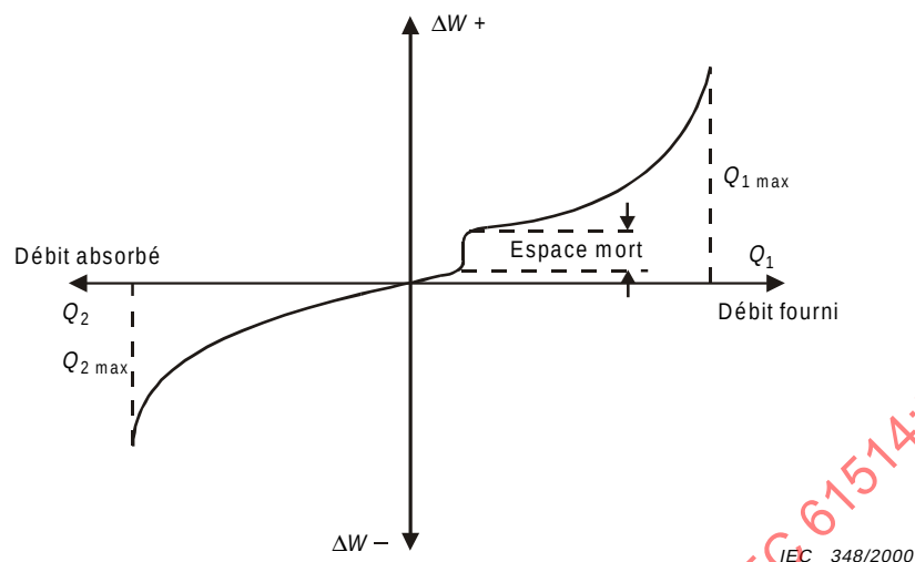
Figure 6 – Caractéristique typique d'un débit d'air
