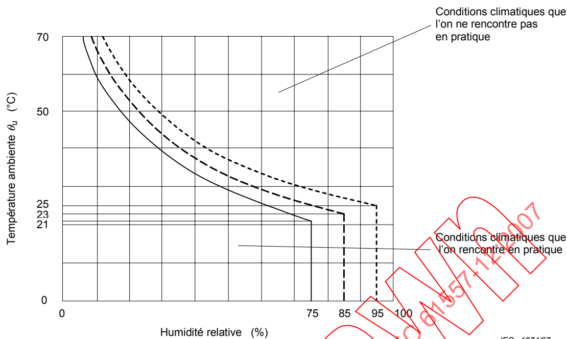
Figure 3 – Relation entre la température de l'air ambiant et l'humidité relative
