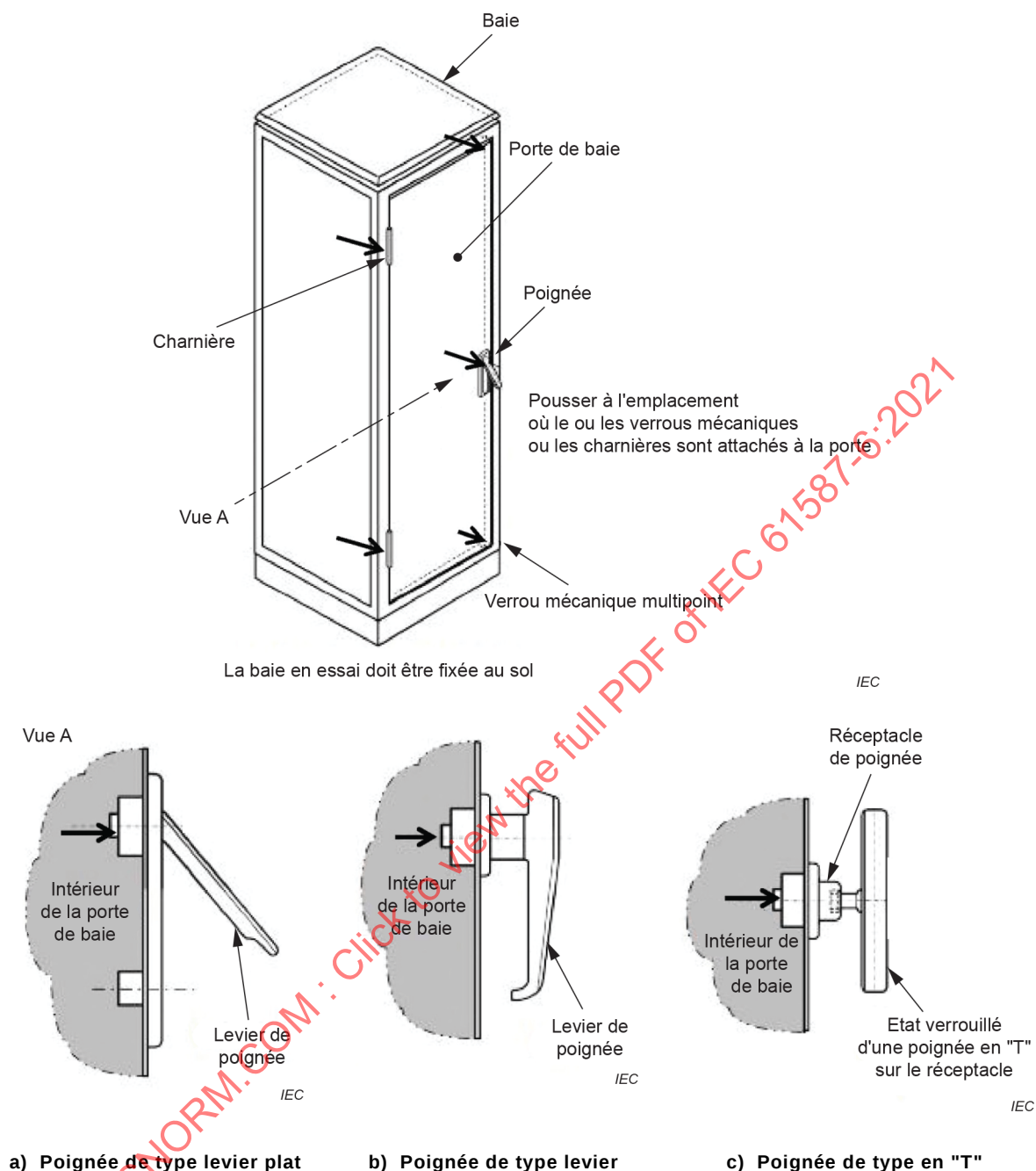
Figure 3 – Essai de charge statique pour charnières et verrous mécaniques
