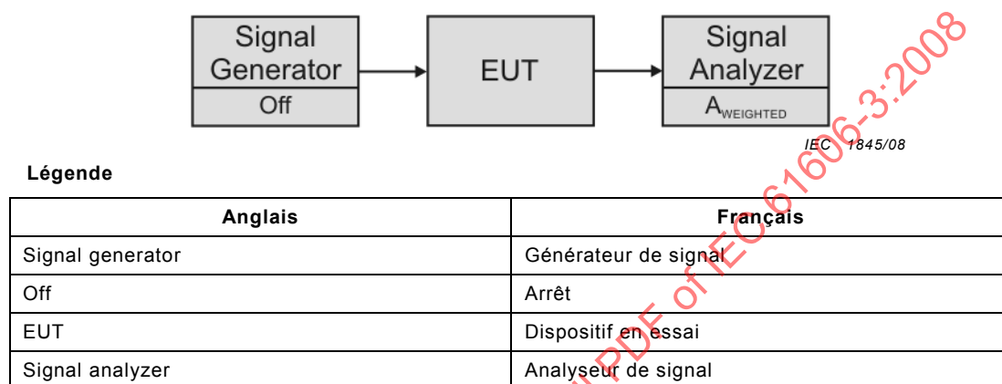
Figure 22 – Méthode du bruit de la voie inactive
