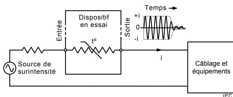
Figure B.5 – Composant limiteur de courant placé en série à deux bornes à fonctionnement thermique (thermistance CTP)
