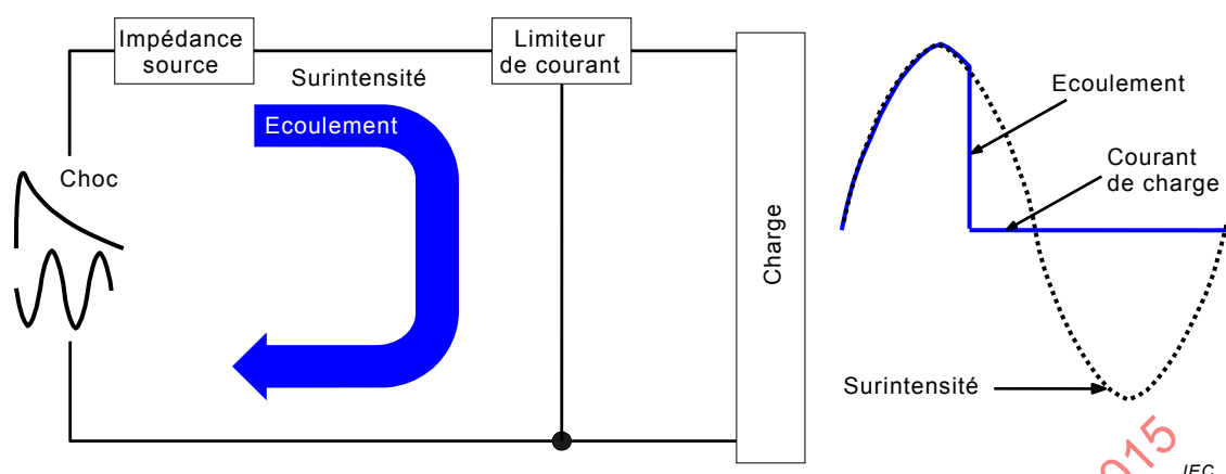
Figure B.2 – Comportement du composant à écoulement de courant
