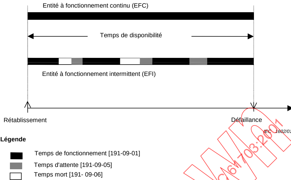
Figure 4 – Comparaison d'un temps de disponibilité pour une EFC et une EFI
