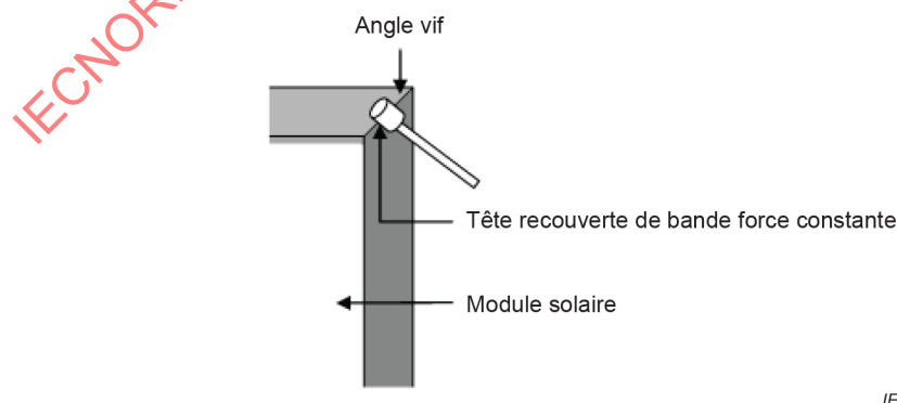
Figure 4 – Position de l'appareillage d'essai
