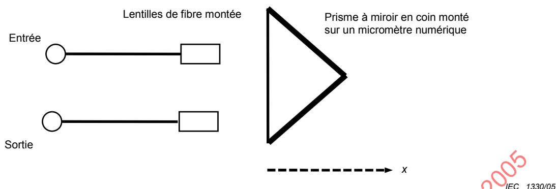
Figure 2 – Artéfact typique de ligne de retard optique pour l'étalonnage du retard d'un l'ensemble d'essai CD
