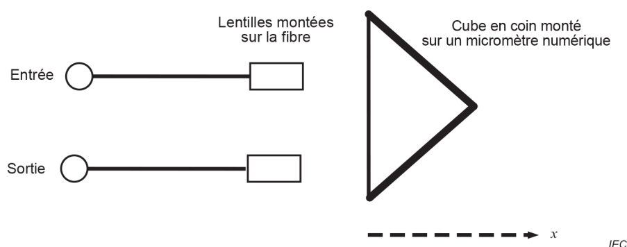
Figure 2 – Artefact typique de ligne de retard optique pour l'étalonnage du retard d'un ensemble d'essai CD
