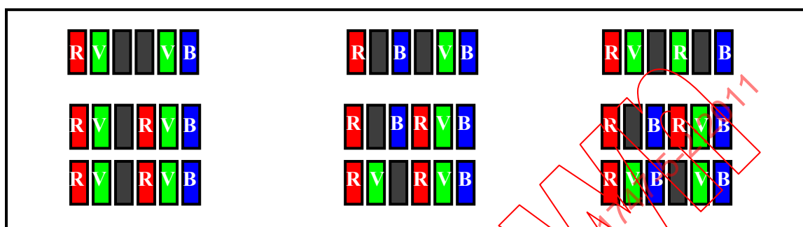
Figure 3 b) – Deux défauts de sous-pixels voisins sombres
