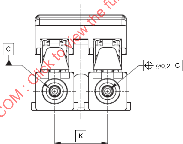
Figure 3 – Interface de connecteurs mâles duplex
