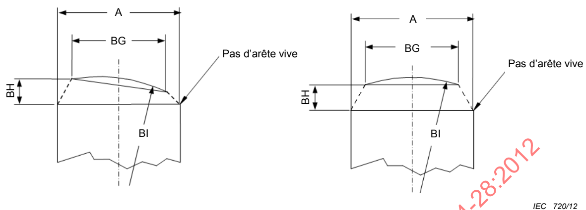
Figure 2 – Géométrie de l'extrémité APC/PC
