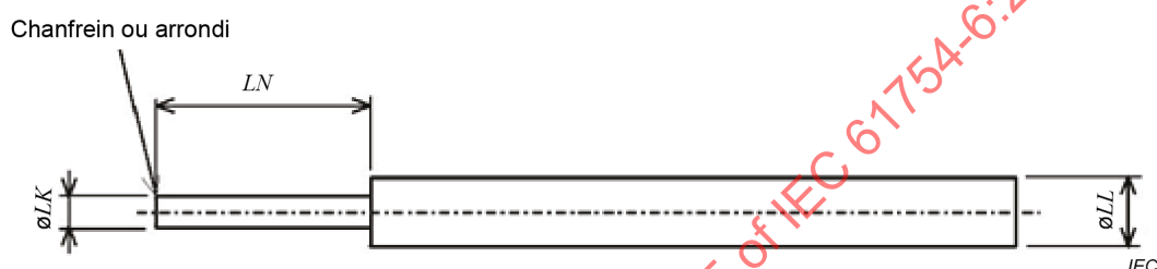
Figure 4 – Broche calibrée pour manchon d'alignement élastique
