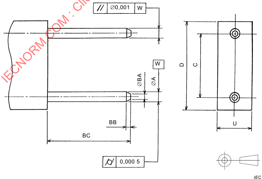
Figure 6 – Calibre pour la fiche
