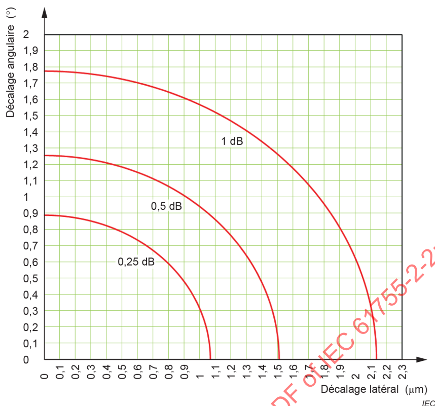
Figure 1 – Décalage latéral et décalage angulaire en fonction de l'affaiblissement, \eta_{\text{combined}} , pour les fibres unimodales de MFD 8,9 \mu\text{m} à 1 310 nm
