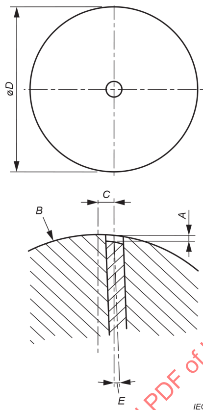
Figure 1 – Dimensions de l'extrémité de la fiche de connecteur
