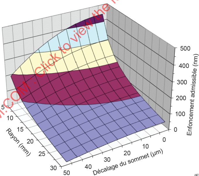
Figure A.1 – Enfoncement admissible en fonction du rayon d'extrémité et du décalage du sommet – Force de contact minimale de 4,9 N
