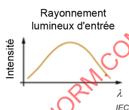
b) Spectre du rayonnement lumineux incident
