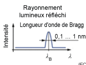
c) Partie réfléchie du spectre du rayonnement lumineux incident
