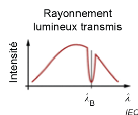
d) Partie transmise du spectre du rayonnement lumineux incident
