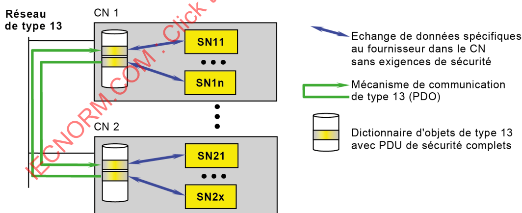
Figure 15 – Transport des SPDO
