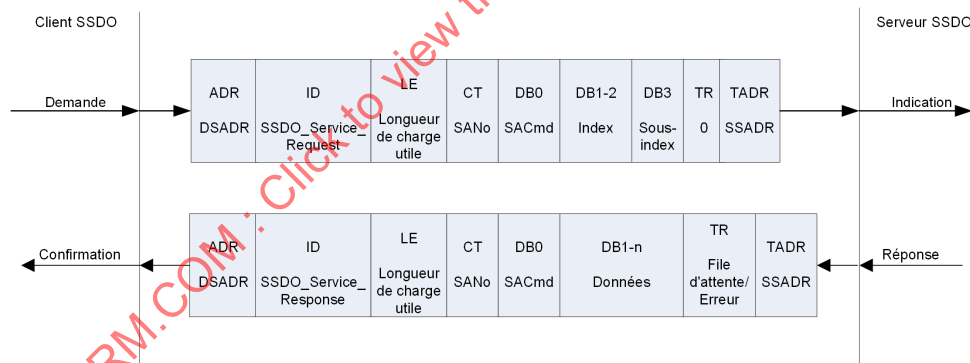
Figure 37 – Protocole Segmenter téléchargement amont SSDO avec préchargement
