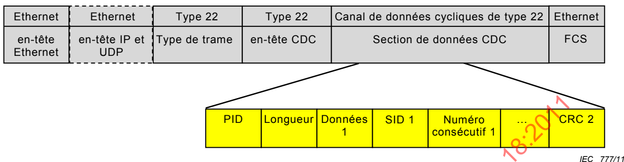
Figure 10 – PDU de sécurité pour le protocole FSCP 18/1 intégrée dans une section de données CDC de type 22
