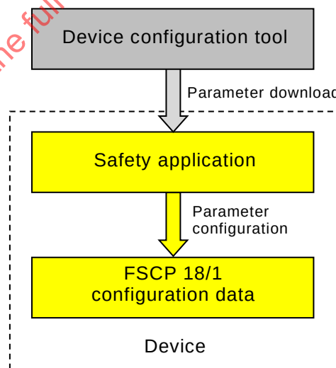
Figure 15 – Parameter handling
