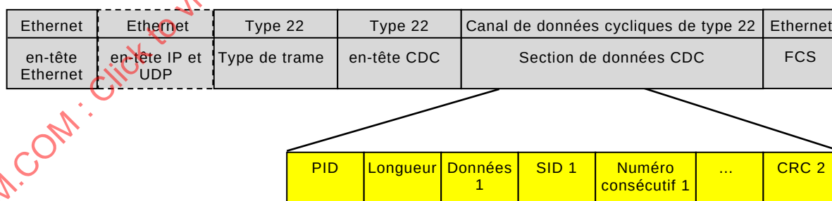
Figure 10 – PDU de sécurité pour le protocole FSCP 18/1 intégrée dans une section de données CDC de type 22
