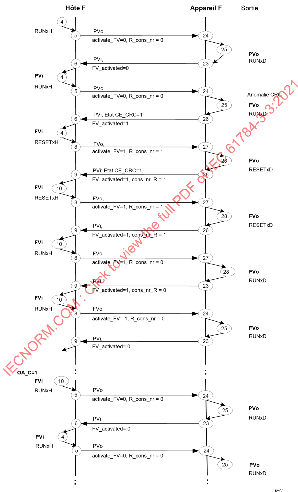
Figure 32 – Interaction lorsque le pilote de l'hôte F reconnaît une erreur CRC
