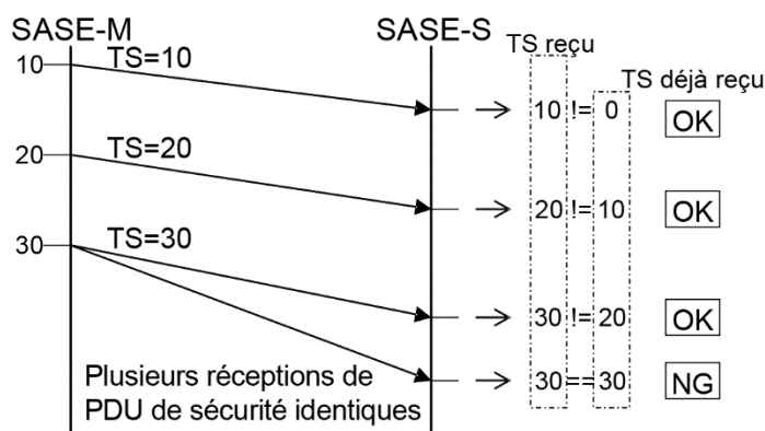
Figure 5 – Détection d'une répétition non prévue
