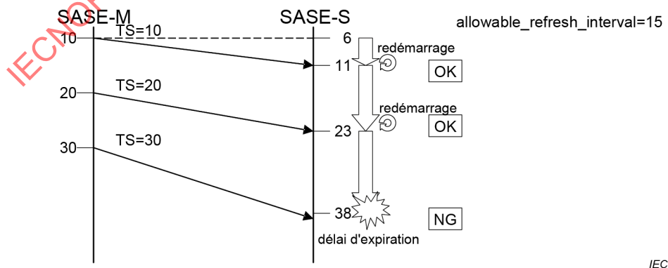
Figure 8 – Détection d'un retard inacceptable par les horodatages
