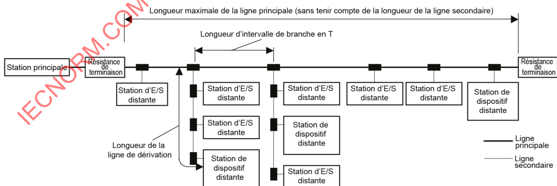
Figure B.2 – Topologie en bus à branche en T
