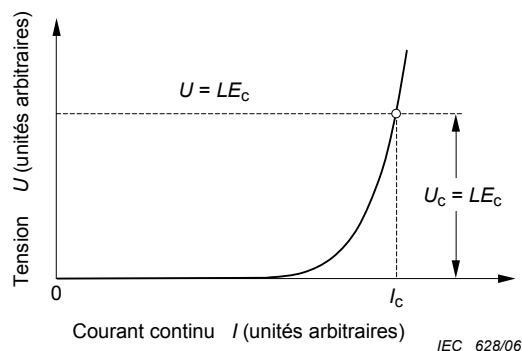
Figure 1a) – Application du critère du champ électrique
