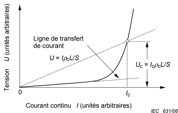
Figure 2b) – Application du critère de résistivité
