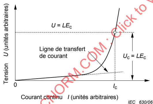
Figure 2a) – Application du critère du champ électrique
