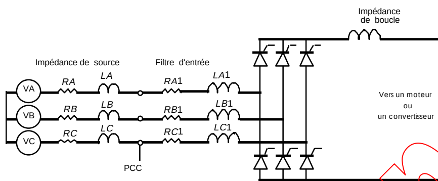
Figure B.1 – Convertisseur à thyristors avec forte inductance dans la boucle de courant continu
