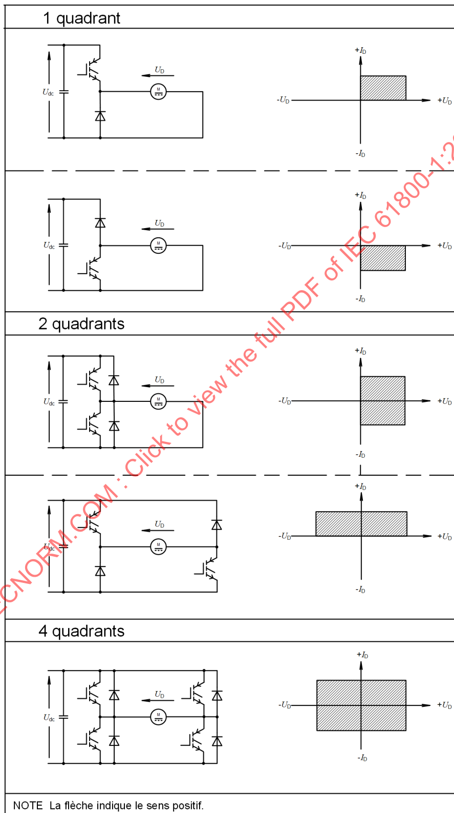
Figure 6 – Principales configurations pour convertisseurs autocommutés (hacheurs)
