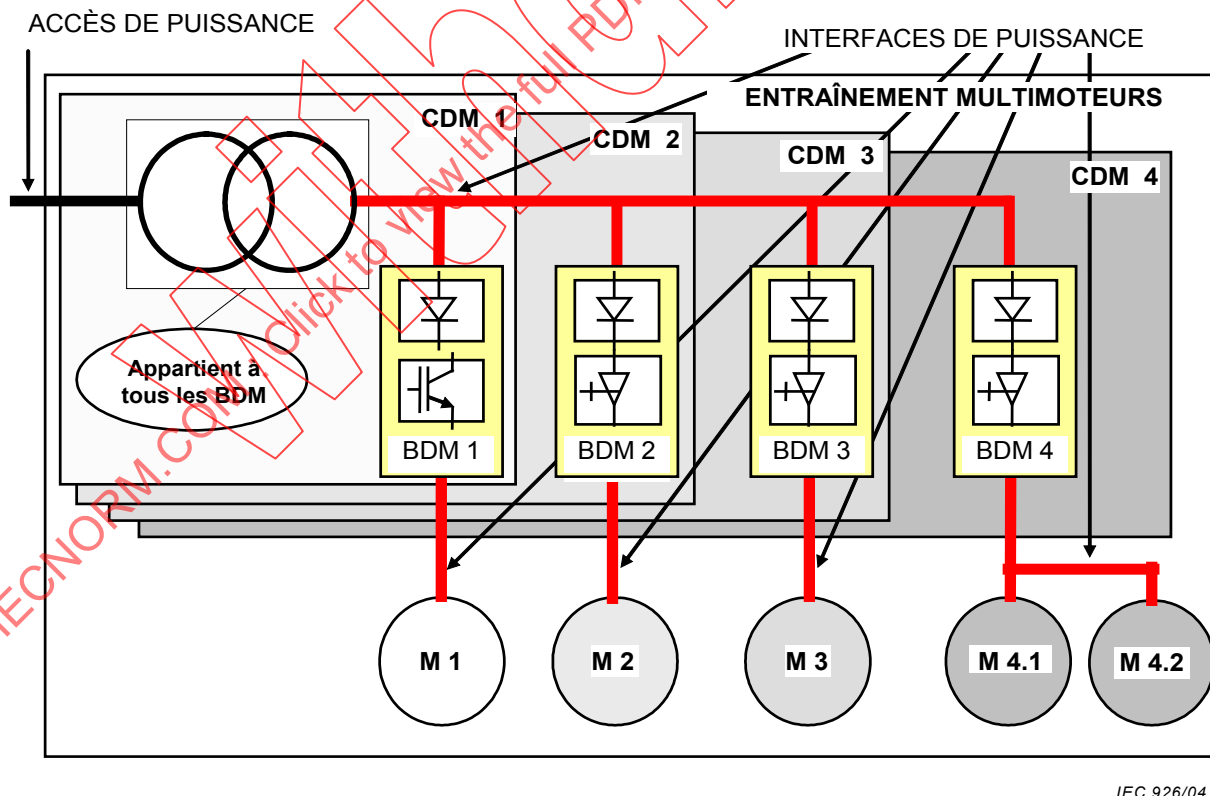
Figure 4 – Interfaces de puissance avec transformateur d'entrée commun
