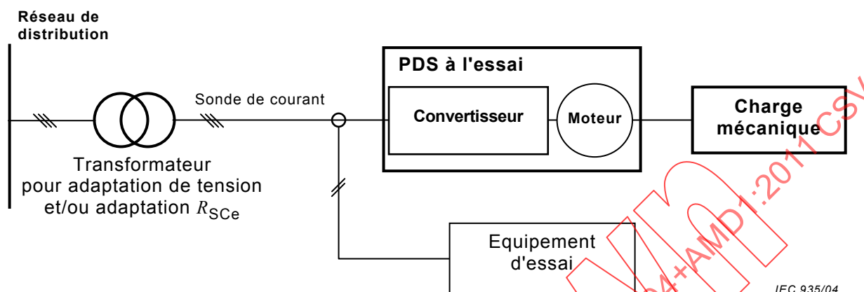
Figure B.6 – Configuration d'essai avec une charge mécanique
