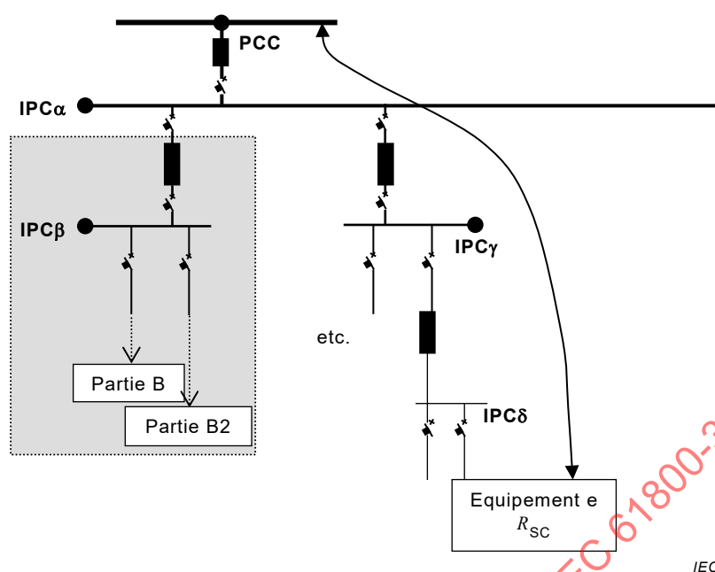
Figure B.3 – PCC, IPC, rapport des courants de l'installation et R_{SC}
