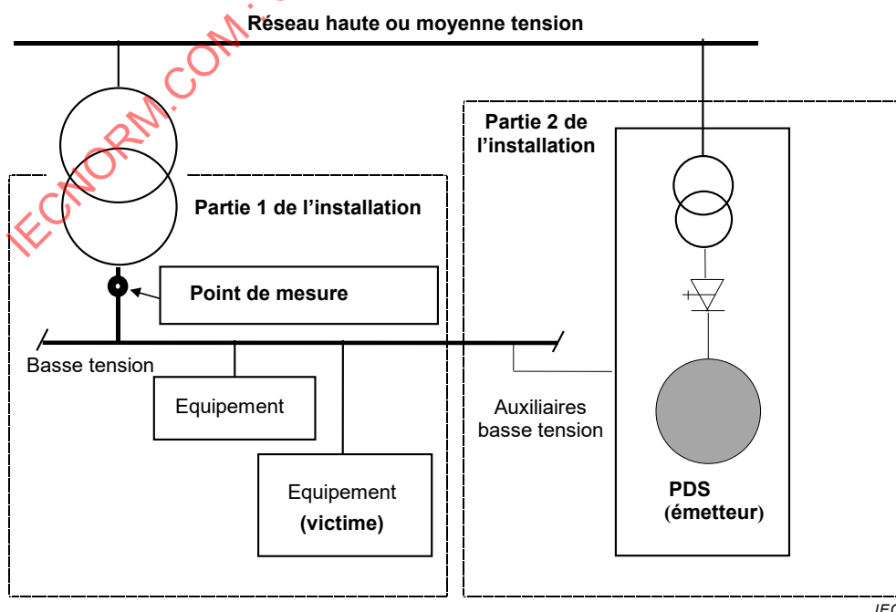
Figure 9 – Propagation des perturbations dans une installation avec un PDS de tension assignée > 1 000 V
