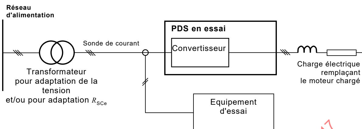
Figure B.6 – Configuration d'essai avec une charge électrique remplaçant le moteur chargé
