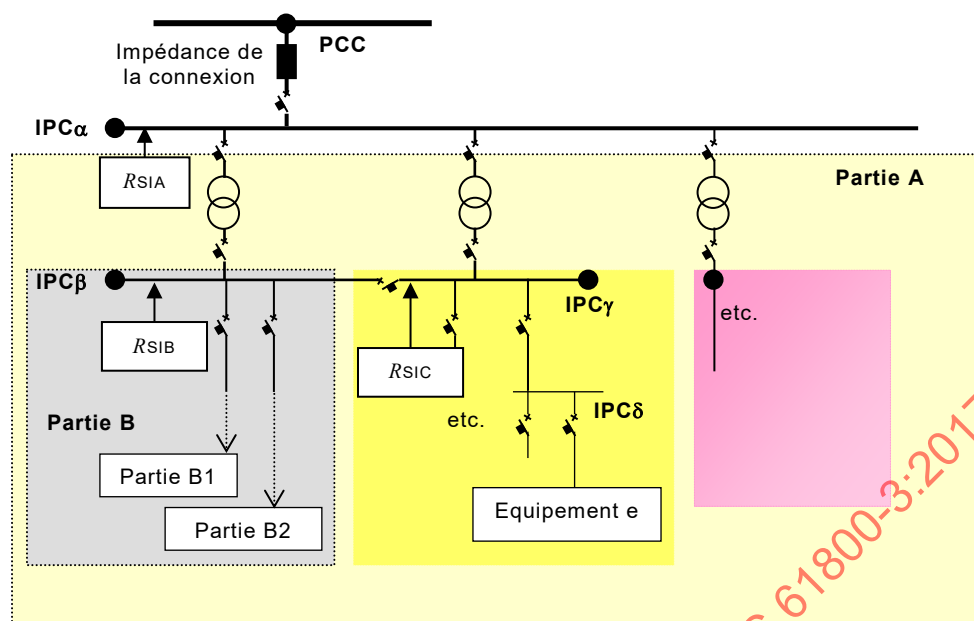
Figure B.2 – PCC, IPC, rapport des courants de l'installation et R_{SI}
