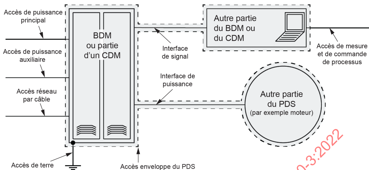
Figure 3 – Interfaces internes d'un PDS et exemples d'accès
