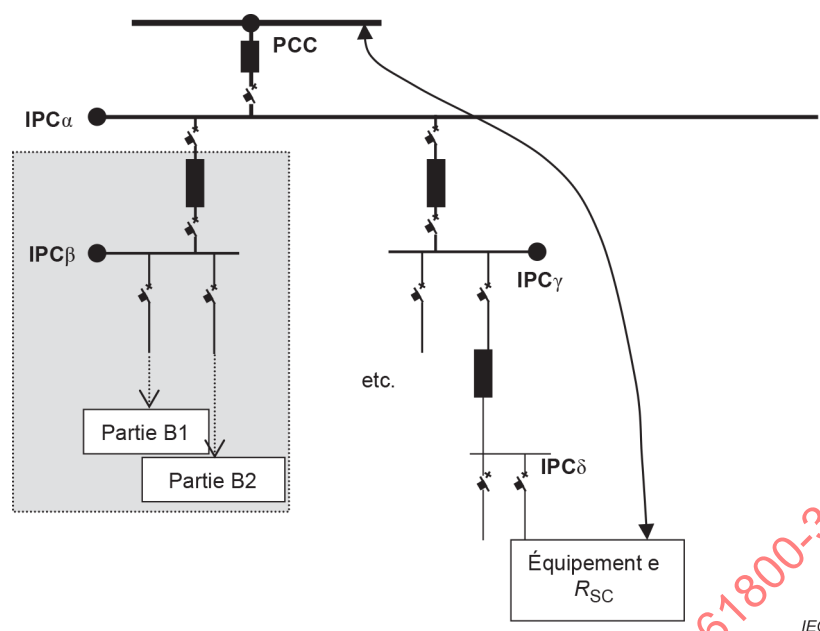
Figure B.3 – PCC, IPC, rapports de courant de l'installation et R_{SC}
