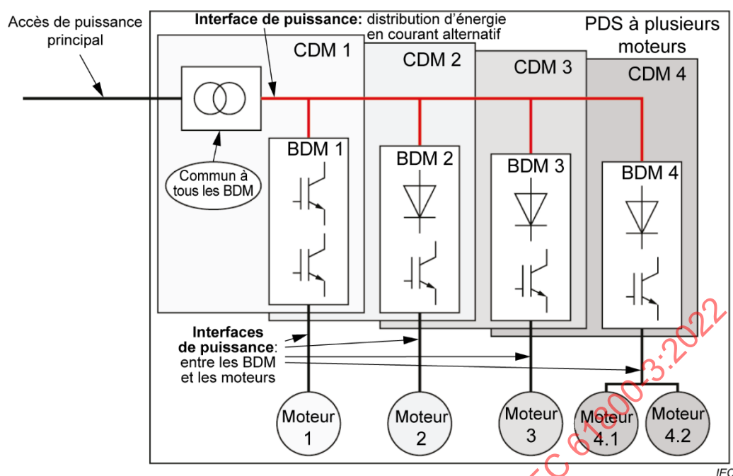
Figure 6 – Interfaces de puissance avec transformateur d'entrée commun
