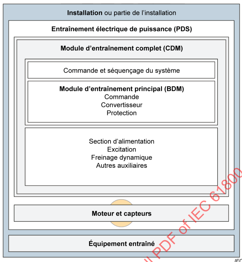
Figure 1 – Contenu du PDS et de son installation
