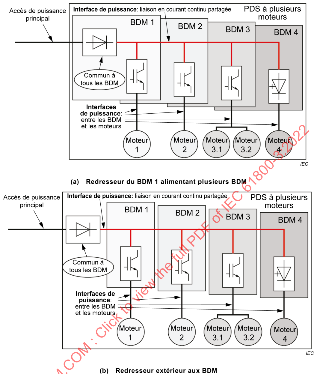
Figure 5 – Interfaces de puissance d'un PDS avec liaison en courant continu commune
