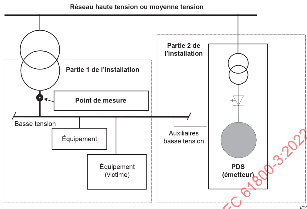
Figure 12 – Propagation des perturbations dans une installation avec un EUT de tension assignée > 1 000 V
