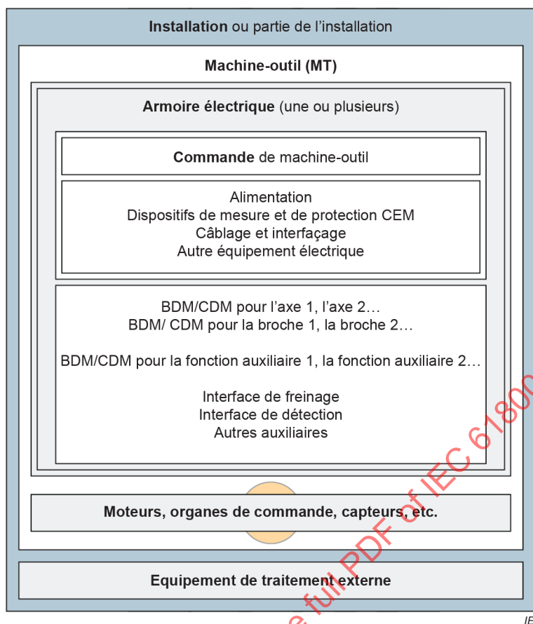
Figure 2 – Contenu de la MT et de son installation
