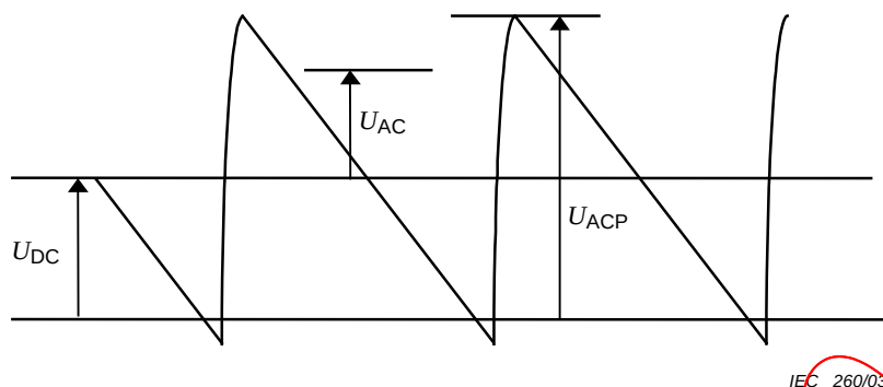
Figure 4 – Forme d'onde typique d'une tension de fonctionnement pulsatoire
