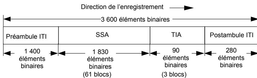
Figure 32 – Structure du secteur de l'information ITI
