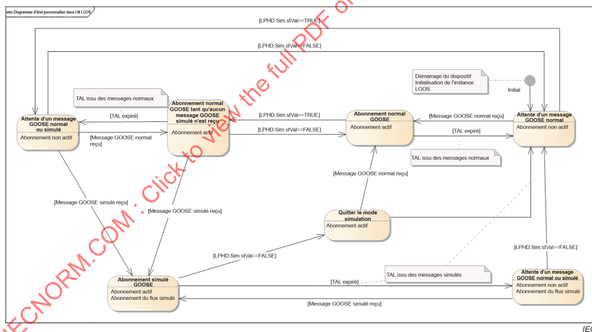
Figure 80 – Diagramme d'états de surveillance d'un abonnement GOOSE
