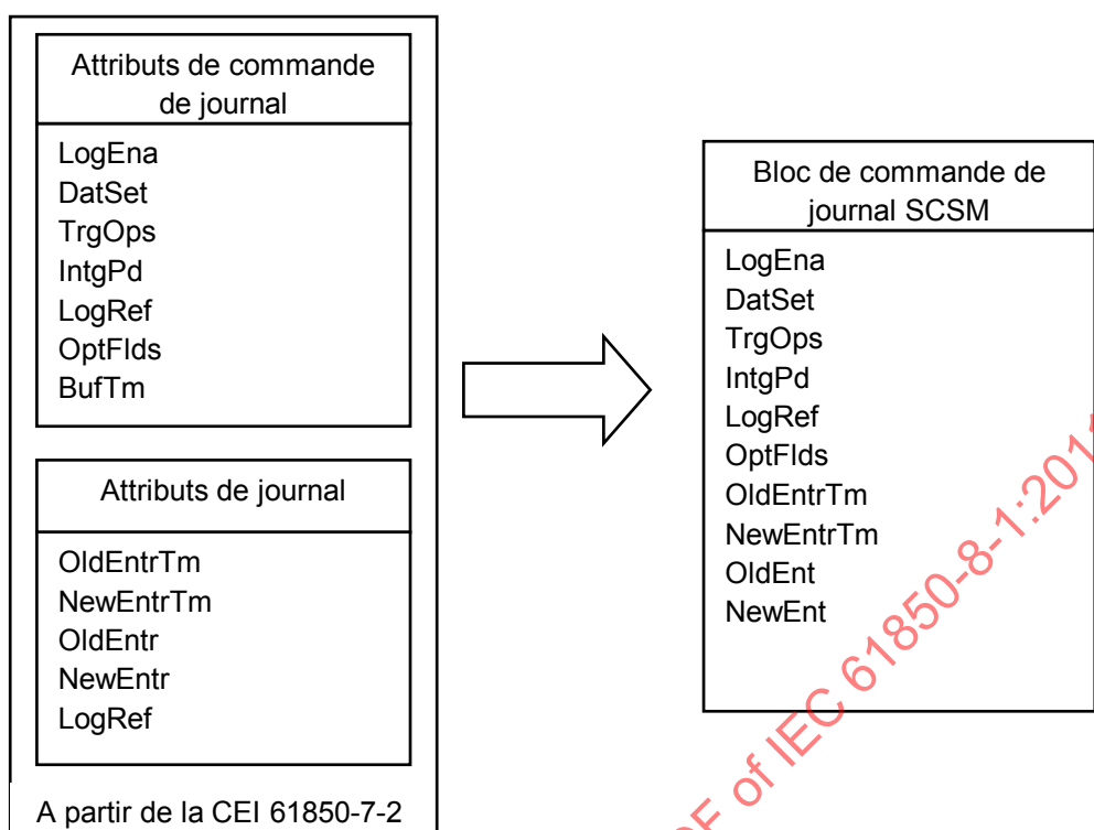
Figure 5 – Relation des attributs LCB avec les définitions de journal (log) de la CEI 61850-7-2
