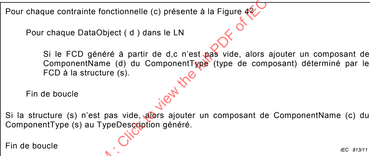
Figure 3 – Algorithme pour la mise en correspondance de nœud logique
