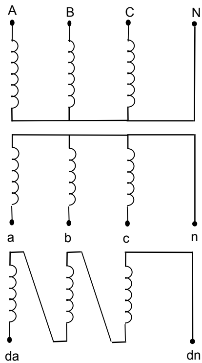
Figure 310 – Transformateur triphasé avec enroulement de tension résiduelle
