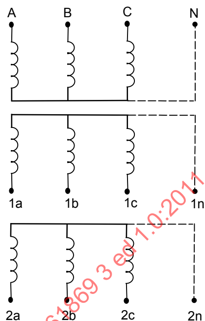
Figure 305 – Ensemble triphasé avec deux circuits secondaires
