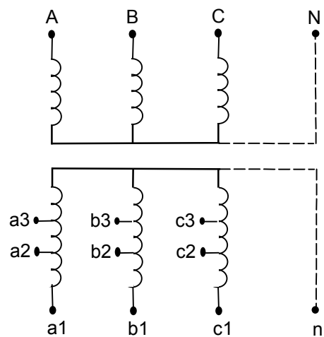
Figure 307 – Ensemble triphasé avec un circuit secondaire à prises multiples
