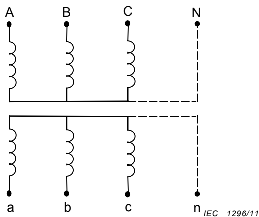
Figure 303 – Ensemble triphasé avec un seul circuit secondaire
