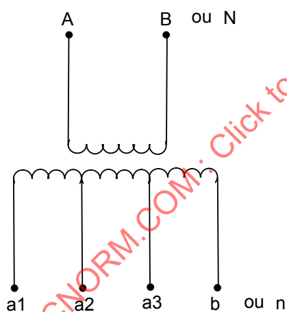
Figure 306 – Transformateur monophasé avec un circuit secondaire à prises multiples
