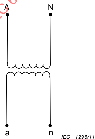
Figure 302 – Transformateur monophasé avec une borne primaire neutre à isolement réduit et un seul circuit secondaire
