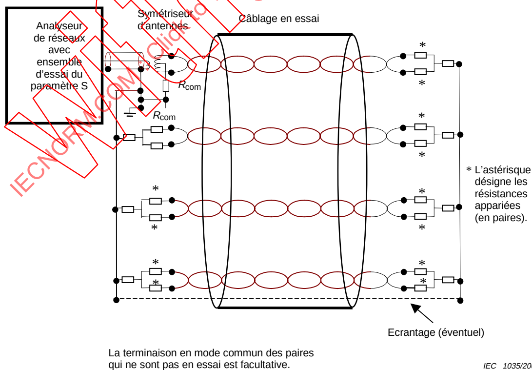
Figure 8 – Configuration d'essai des pertes par réflexion
