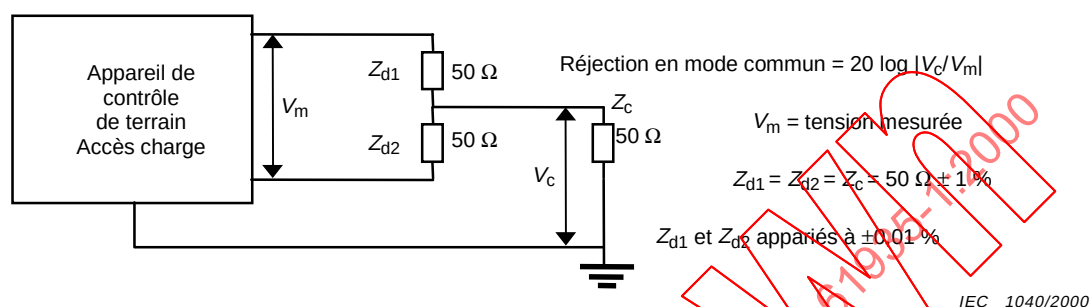
Figure 13 – Schéma fonctionnel de mesure de la réjection en mode commun
